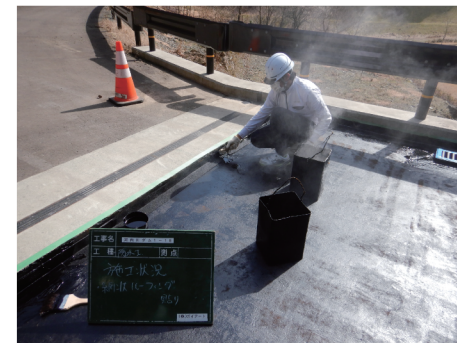
④網状ルーフィング貼り
