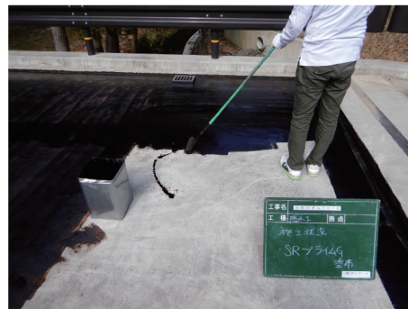
③SRプライムG塗布
