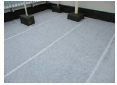
③テクノシート敷設作業
